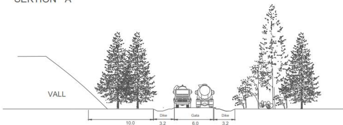
Fig 7. Förslag till breddning av angränsande väg för att hantera ökad tung trafik.
