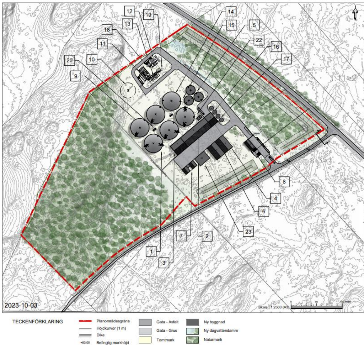
Fig 4. Placering av anläggningens komponenter. Beskrivning av komponenter återfinns i tabell 2.
