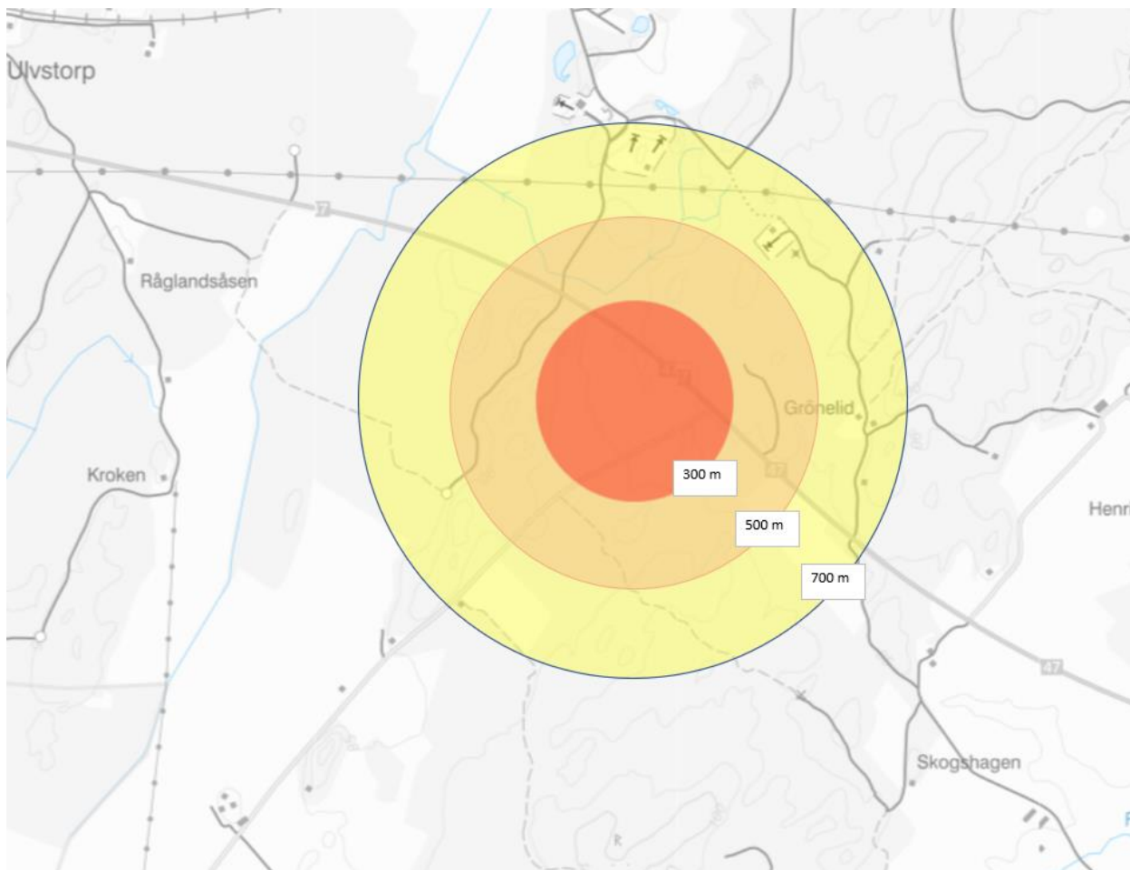
Fig 10. Konsekvensavstånd för en BLEVE. Där de 700 m meter närmast olyckan kan utsättas för över 6 kW/m 2 . Där 6 kW/m 2 kan ge andra gradens brännskador vid 60 sekunders exponering och över 10 kW/m 2 är dödligt inom 60 sekunders exponering. [19]
