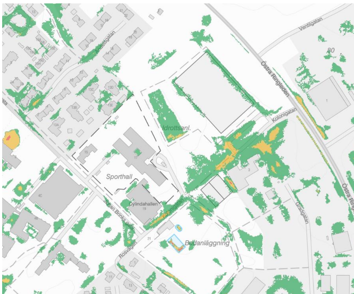
2Bilden ovan är ett skärmdump från Scalgo som redovisar hur ett skyfall påverkar planområdet och angränsande bebyggelse idag. Flödena är beräknade utifrån ett 100 års regn motsvarande 50 millimeter. Grönt 0-20cm, gult 20-50cm, rött >50cm.
